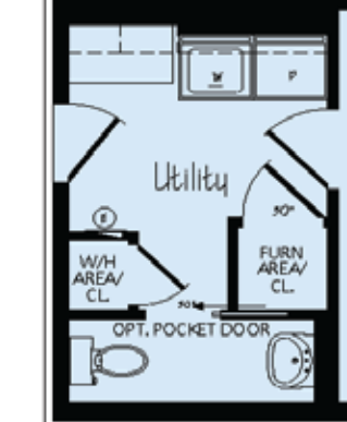
Optional Half Bath
