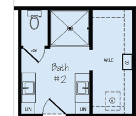
Optional Bath #2 Shower 'Opt'
